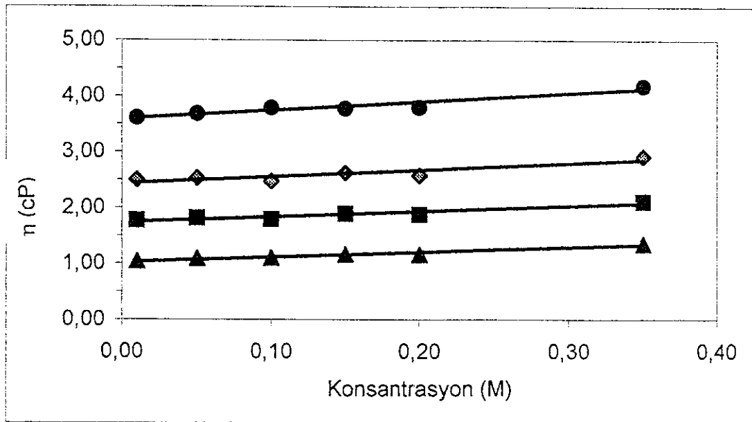
Şekil 3.14. SA çözeltileri için tüm sıcaklıklarda viskozite-konsantrasyon grafiği ●20°C ◆30°C ■40°C ▲60°C
