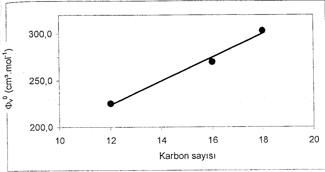
Şekil 3.10. \Phi_v^0 in 40 °C' de karbon sayısı ile değişimi
