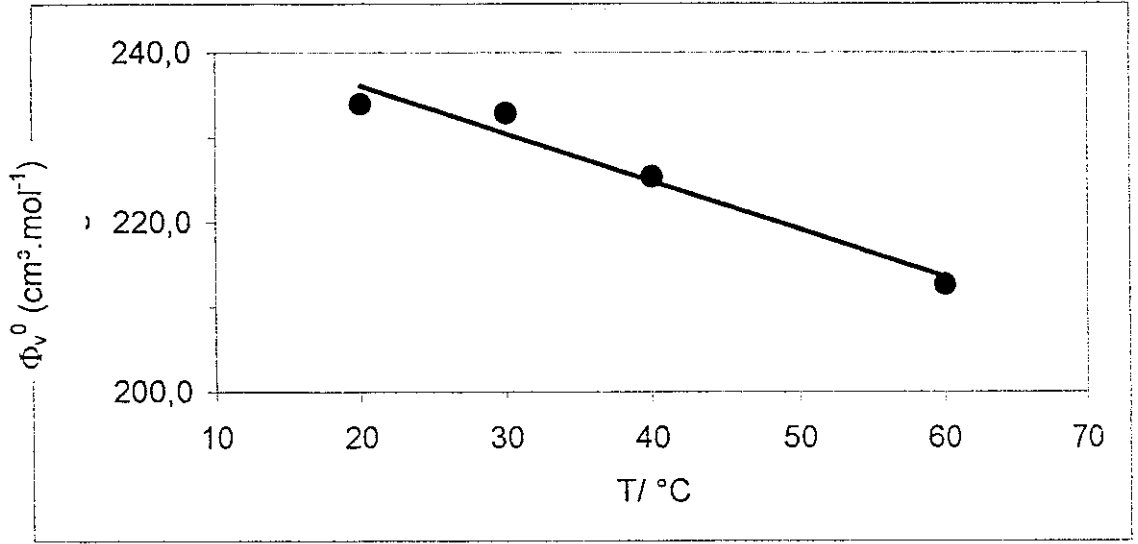
Şekil 3.4. LA için \Phi_v^0 in sıcaklıkla değişim grafiği
