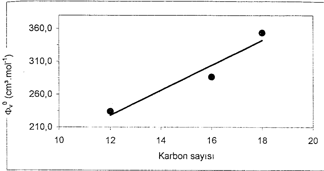
Şekil 3.8. \Phi_v^0 in 20 °C' de karbon sayısı ile değişimi
