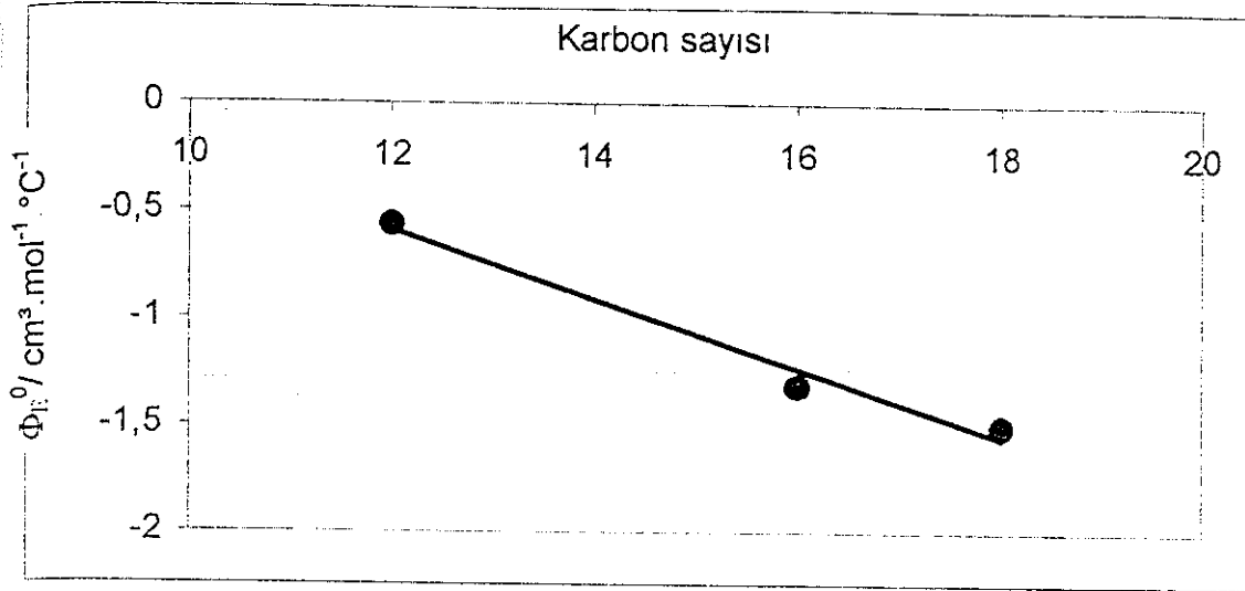
Şekil 3.7. \Phi_E^0 'ın karbon sayısı ile değişimi
