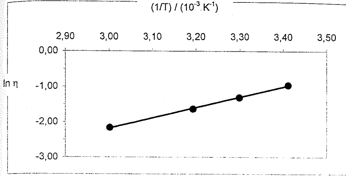
Şekil 3.15. 0,35M LA çözeltisi için \ln \eta - 1/T grafiği
