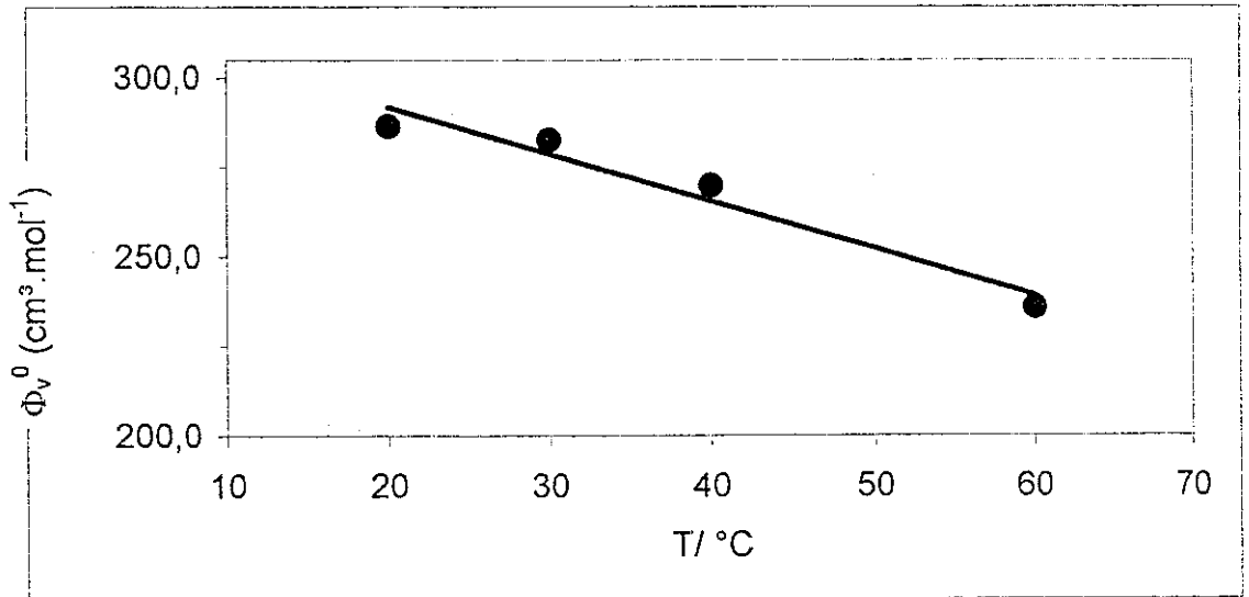
Şekil 3.5. PA için \Phi_v^0 in sıcaklıkla değişim grafiği
