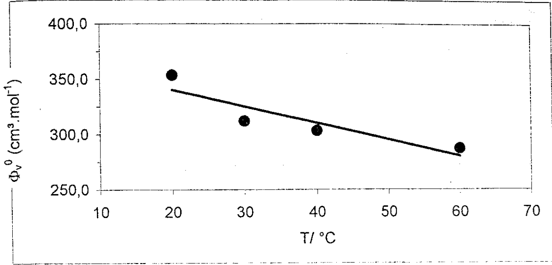
Şekil 3.6. SA için \Phi_V^0 in sıcaklıkla değişim grafiği
