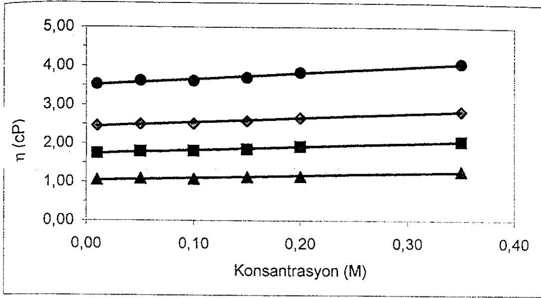
Şekil 3.13. PA çözeltileri için tüm sıcaklıklarda viskozite-konsantrasyon grafiği ●20°C ◆30°C ■40°C ▲60°C
