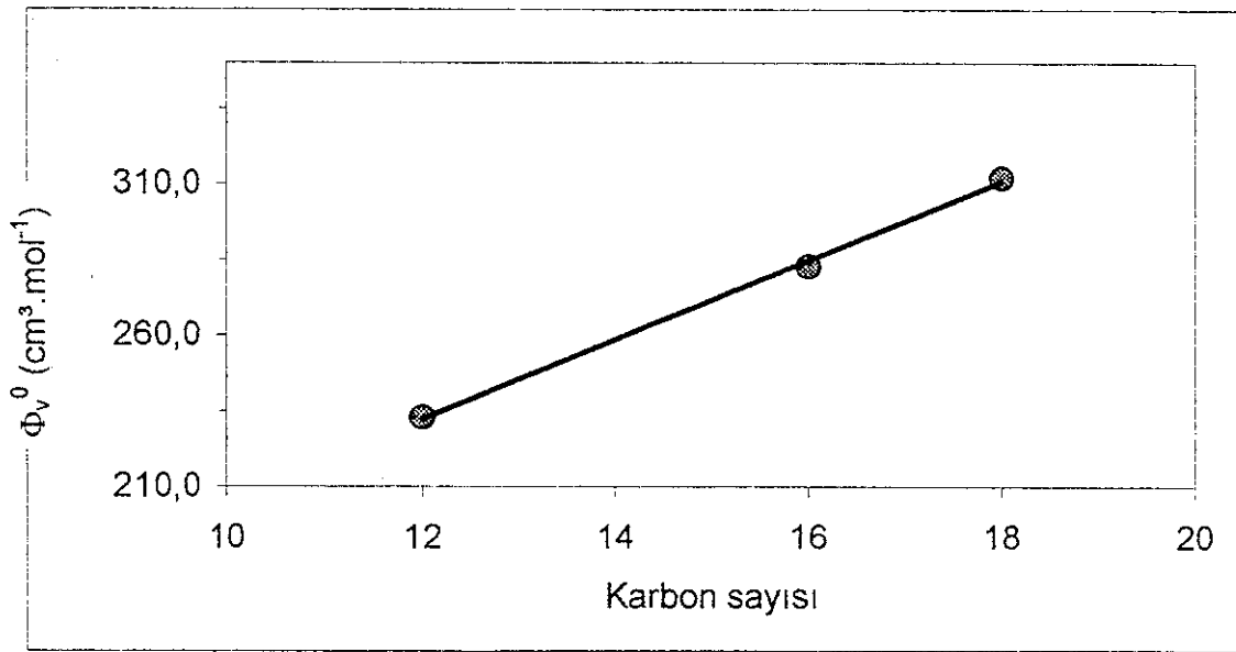
Şekil 3.9. \Phi_v^0 in 30 °C' de karbon sayısı ile değişimi
