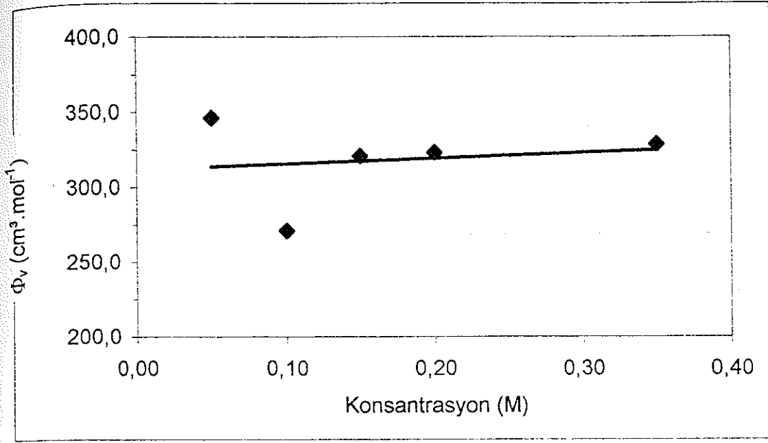
Şekil 3.3.b. SA için 30 °C' de görünür molar hacim-konsantrasyon grafiği
