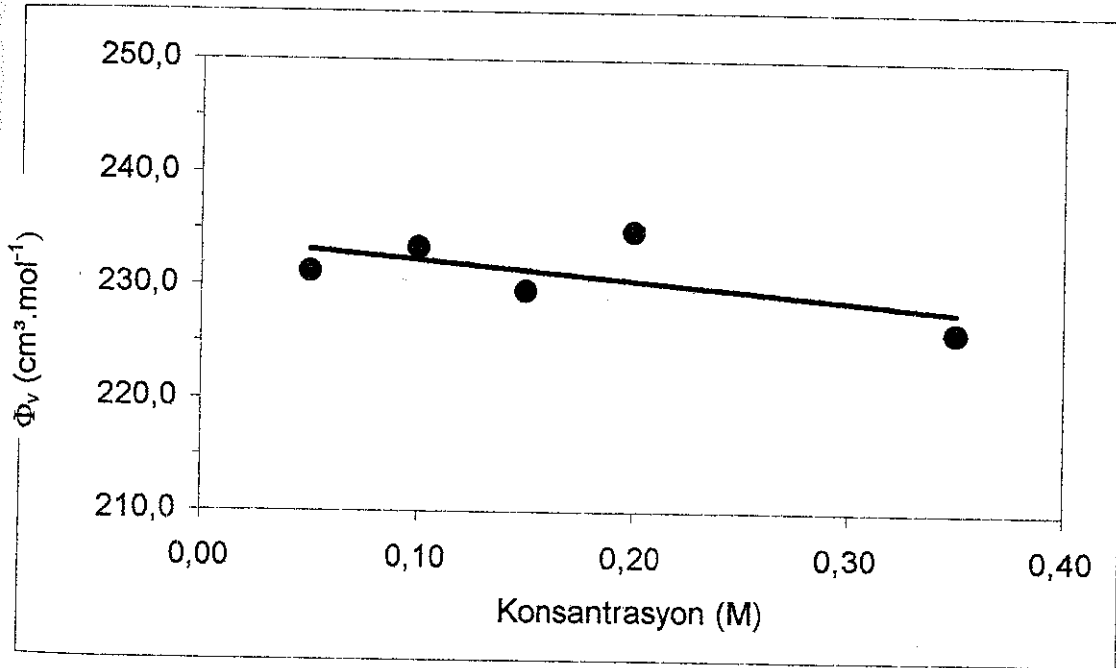
Şekil 3.1.a. LA için 20 °C' de görünür molar hacim-konsantrasyon grafiği
