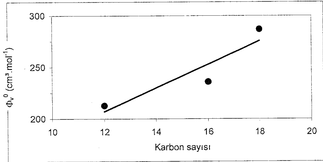
Şekil 3.11. \Phi_v^0 in 60 °C' de karbon sayısı ile değişimi
