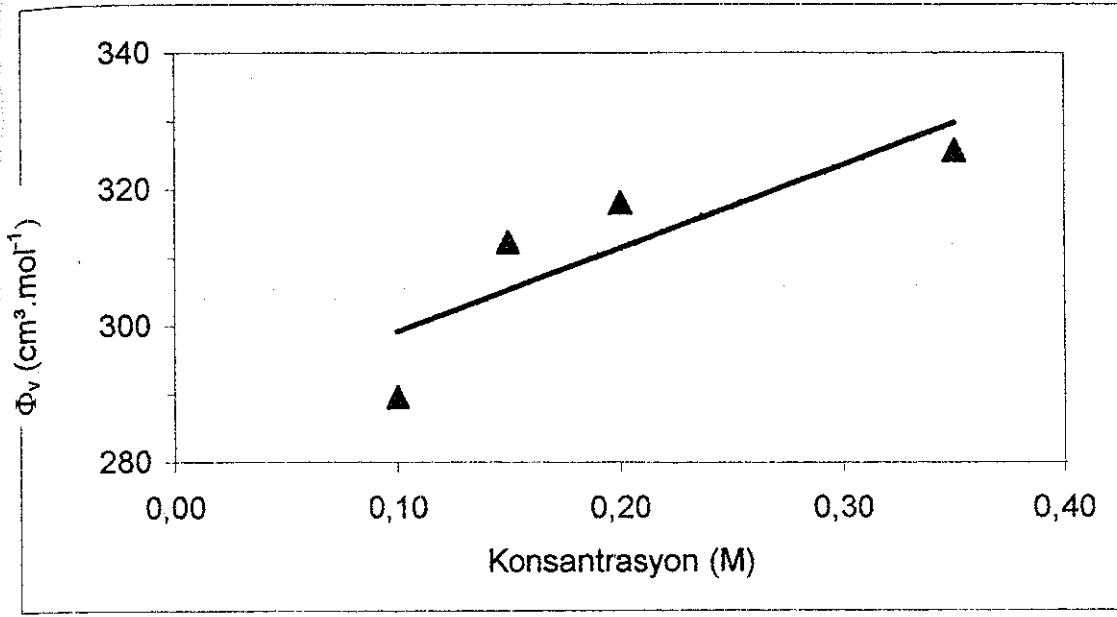
Şekil 3.3.d. SA için 60 °C' de görünür molar hacim-konsantrasyon grafiği
