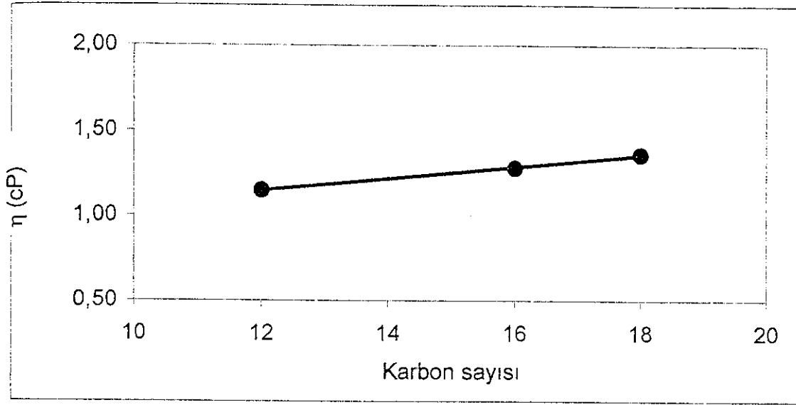
Şekil 3.16. 0,35M çözelti derişimi ve 60 °C için viskozite değerlerinin yağ asidi zincirindeki karbon sayısı ile değışim grafiğı
