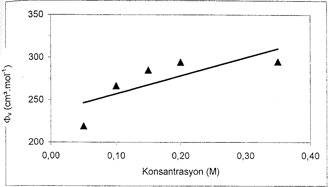
Şekil 3.2.d. PA için 60 °C' de görünür molar hacim-konsantrasyon grafiği
