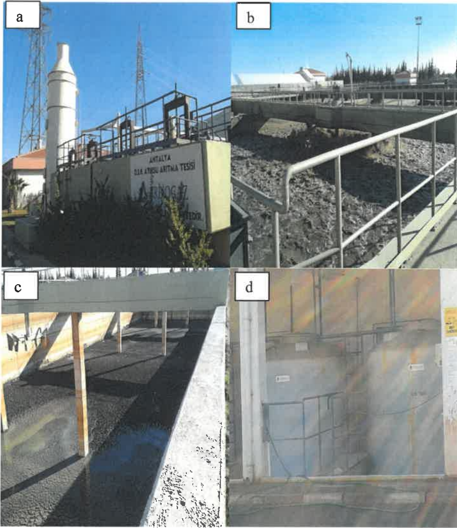
Şekil 2.3. a) Arbiogaz arıtma tesisi, b) Atık su toplama havuzu, c) Çamur kurutma havuzu, d) FeCl 3 asit tankları
