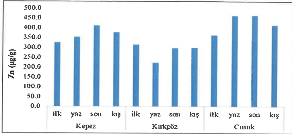
Şekil 4.27. Örnekleme İstasyonlarının Mevsimler Ve İstasyonlara Göre Zn (Çinko) Konsantrasyonları
