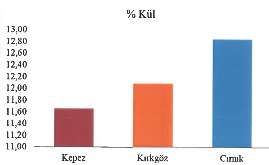
Şekil 4.9. Avlanan Balıkların Vücut Bileşimindeki % Kül Oranının İstasyonlara Göre Değişimi
