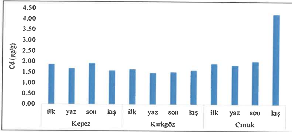
Şekil 4.13. Örnekleme İstasyonlarının Mevsimler ve İstasyonlara Göre Cd (Kadmium) Konsantrasyonları
