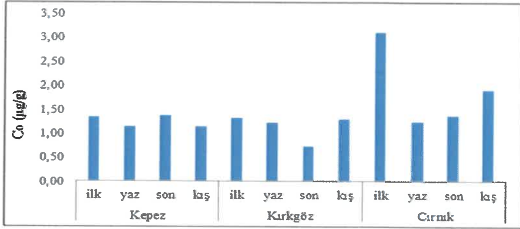
Şekil 4.15. Örneklem İstasyonlarının Mevsimler Ve İstasyonlara Göre Co Konsantrasyonları
