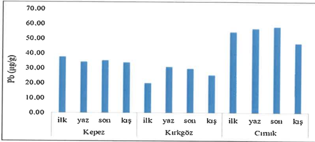
Şekil 4.25. Örnekleme İstasyonlarının Mevsimler ve İstasyonlara Göre Pb (Kurşun) Konsantrasyonları
