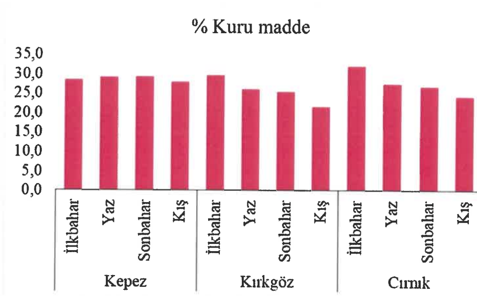
Şekil 4.2. Çiçek Balığının Vücut Bileşiminde % Kuru Madde Oranının İstasyonlardaki Mevsimsel Değişimi.
