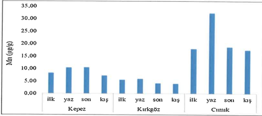
Şekil 4.21. Örnekleme İstasyonlarının Mevsimler ve İstasyonlara Göre Mn (Mangan) Konsantrasyonları
