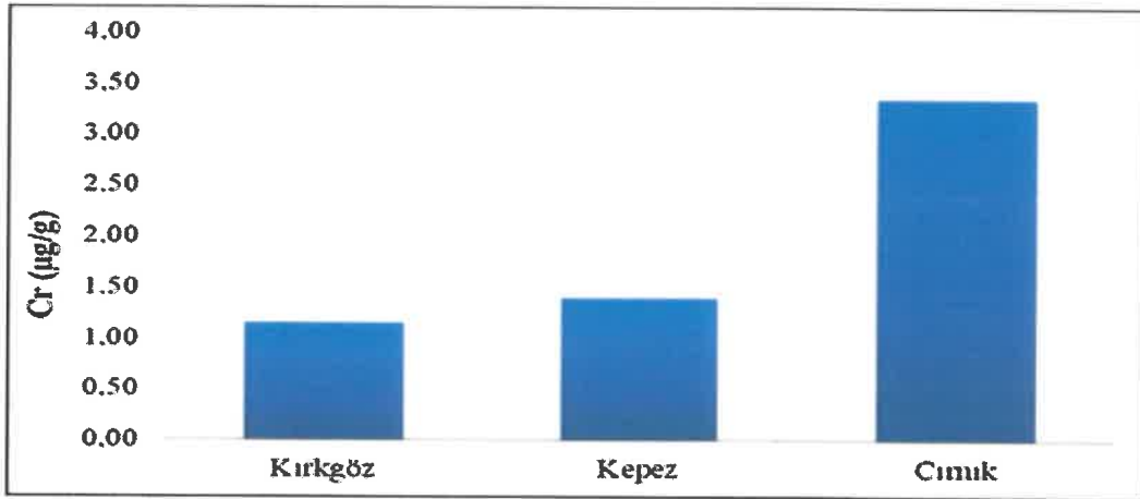
Şekil 4.18. Araştırma İstasyonlarından Örneklenen Balıkların İstasyonlara Göre (Mevsimlerin Ortalaması) Cr Konsantrasyonları
