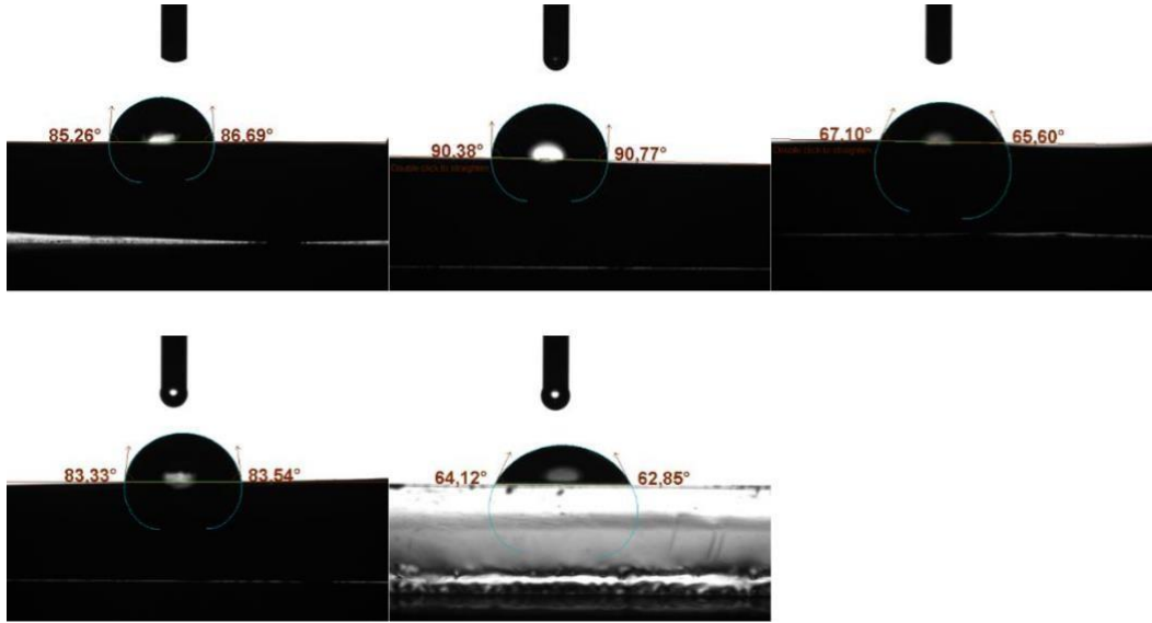
Şekil 4.2.2. Temas açısı ölçümlerinde kullandığımız test örneklerine ait fotoğraflar
