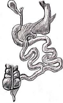
Şekil.2.5. Biliopankreatik Diversiyon ve Duedonal Switch
