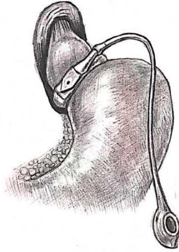
Şekil.2.1. Ayarlanabilir Gastrik Band
