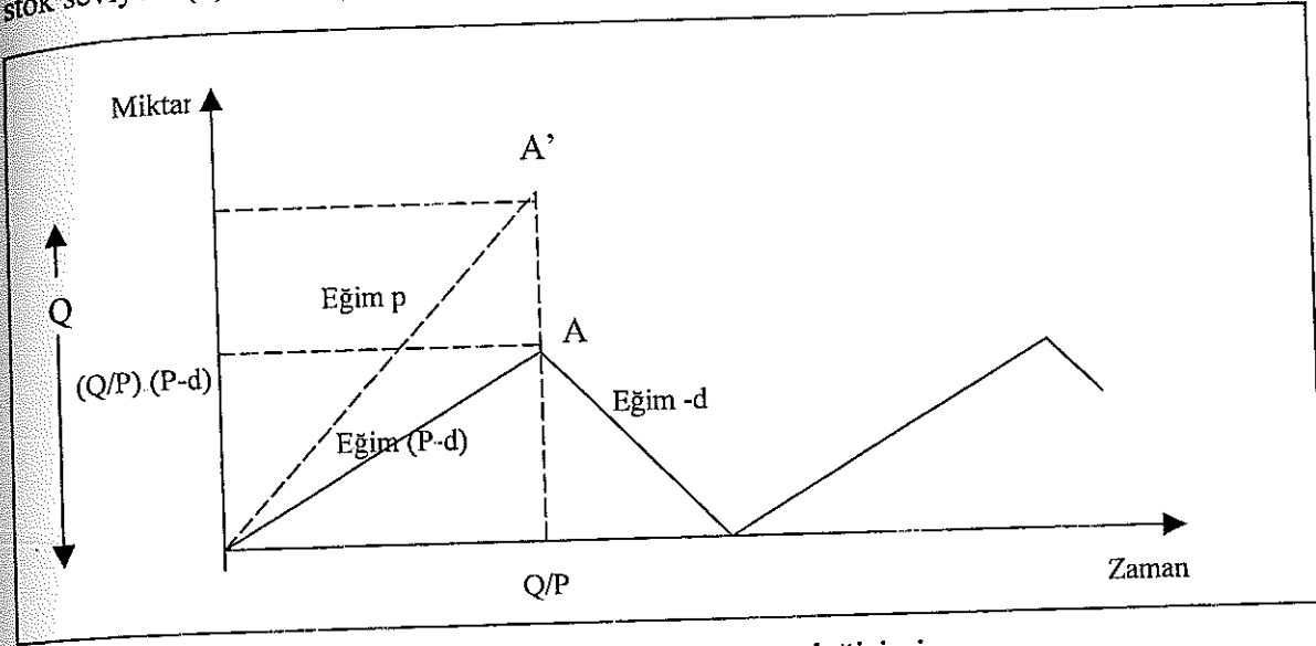
Şekil 4.11. Sürekli tedarik halinde stok miktarı- zaman değişimi
