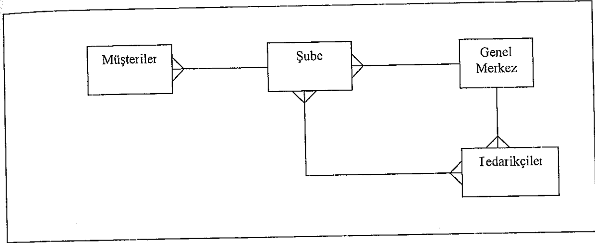
Şekil 5.2 Sisteme İlişkin Veri Yapısı Diyagramı
