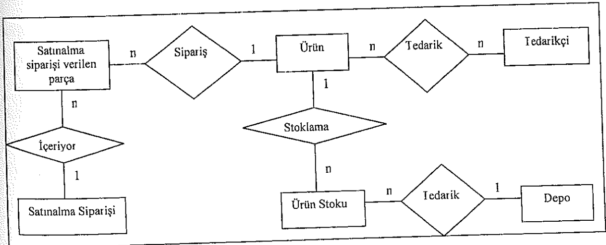
Şekil 3.12. Varlık İlişki Diyagramı
