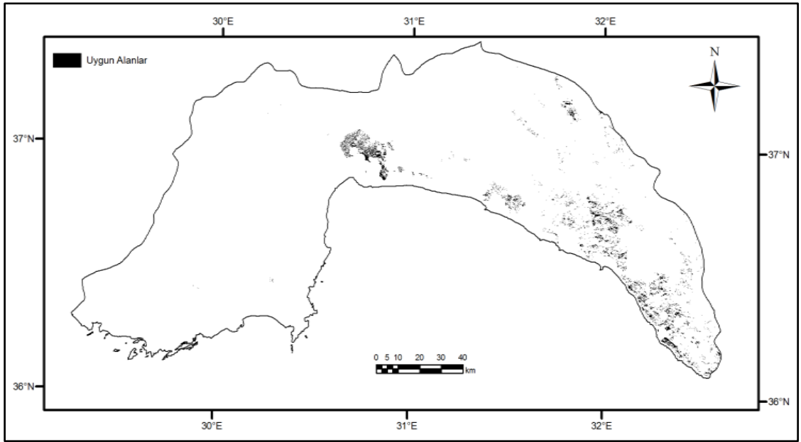
Şekil 3.42. Eşik değeri, ortalama+2*standart sapma’ya göre uygun alanlar
