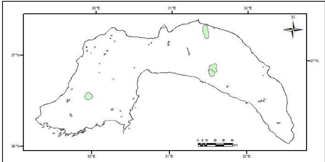
Şekil 3.7. Antalya ili vektör - tampon göller haritası
