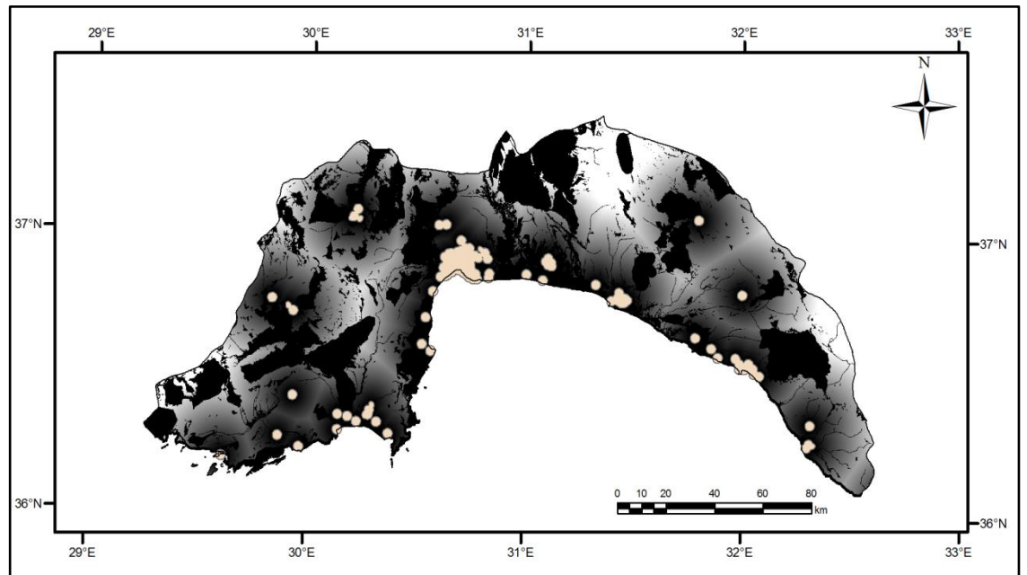
Şekil 3.36. Antalya ili nüfus yoğunluğuna uzaklık verisi
