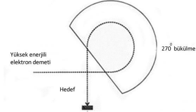
Şekil 2.15: Bükücü mıknatıs 17
