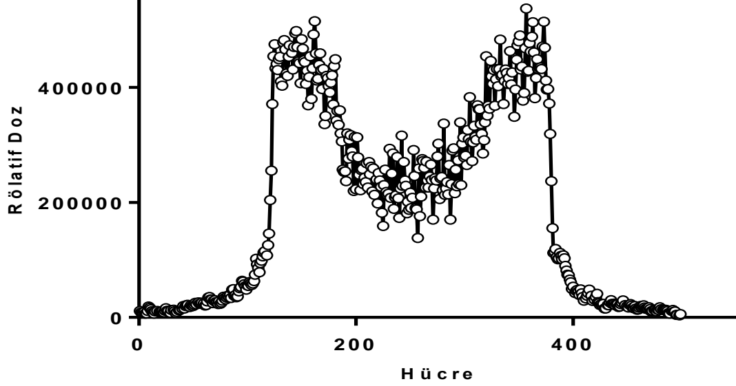
Şekil 3.6: Düzleştirici filtrenin fazla ince olması halinde elde edilen doz profili
