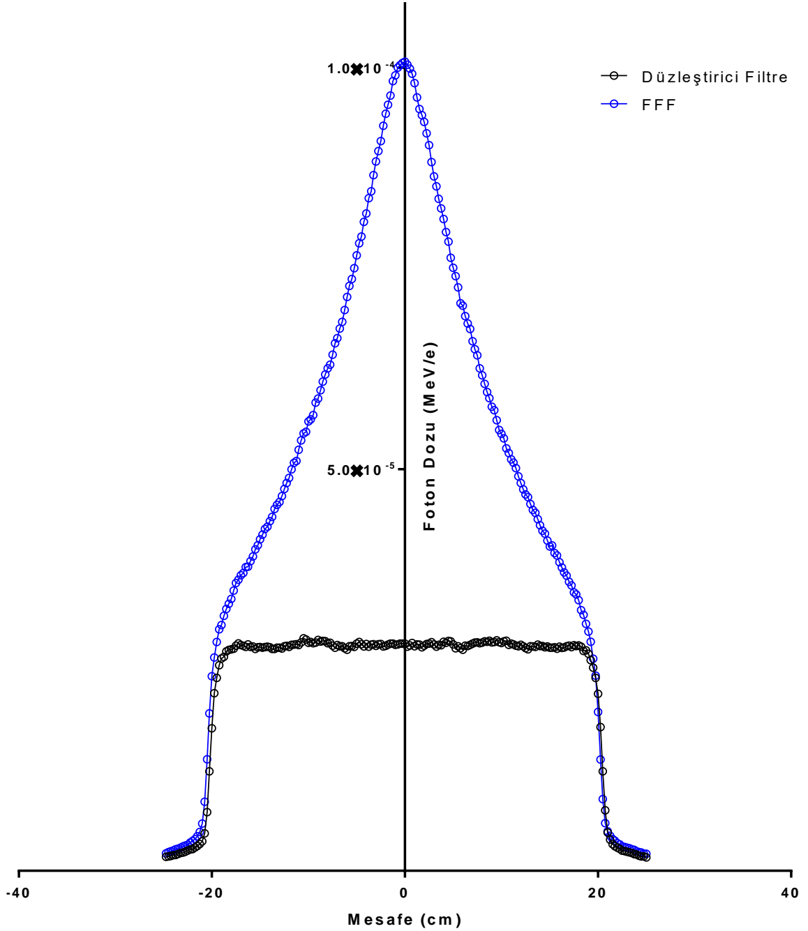
Şekil 4.13: 18 MV foton enerjisi ile 40x40 alan açıklığında filtreli ve filtersiz sistemde birim elektrondan elde edilen doz profili deęerleri
