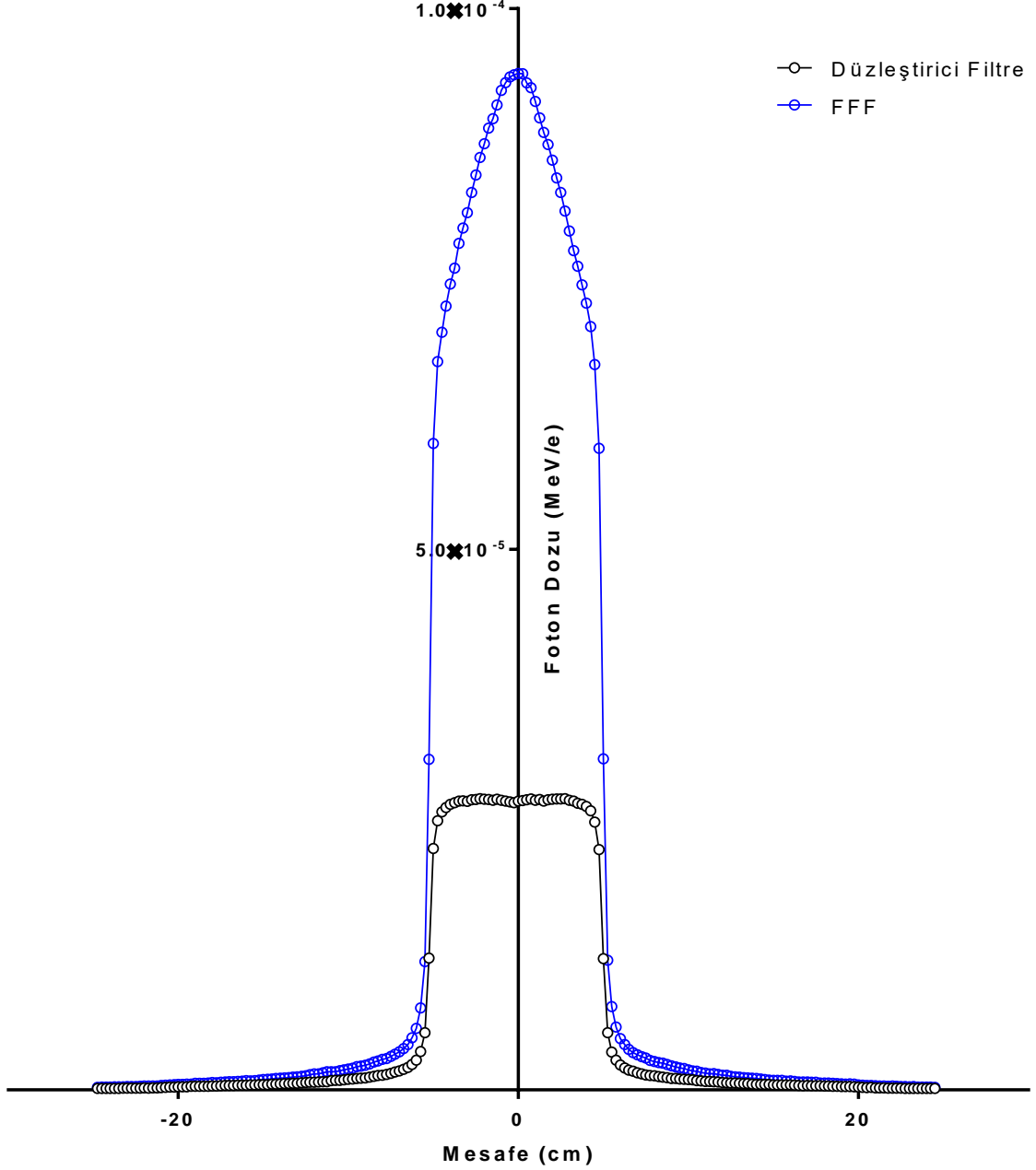
Şekil 4.11: 18 MV foton enerjisi ile 10x10 alan açıklığında filtreli ve filtresiz sistemde birim elektrondan elde edilen doz profili değerleri
