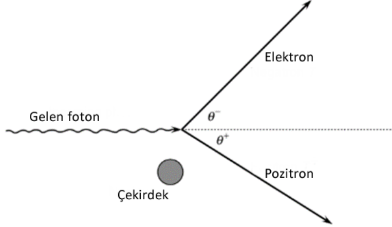
Şekil 2.6: Çift oluşumu 7
