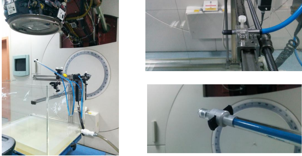
Şekil 3.2: Su Fantomu ve iyon odaları 24
