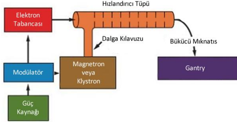
Şekil 2.11: Medikal lineer hızlandırıcı şeması 13
