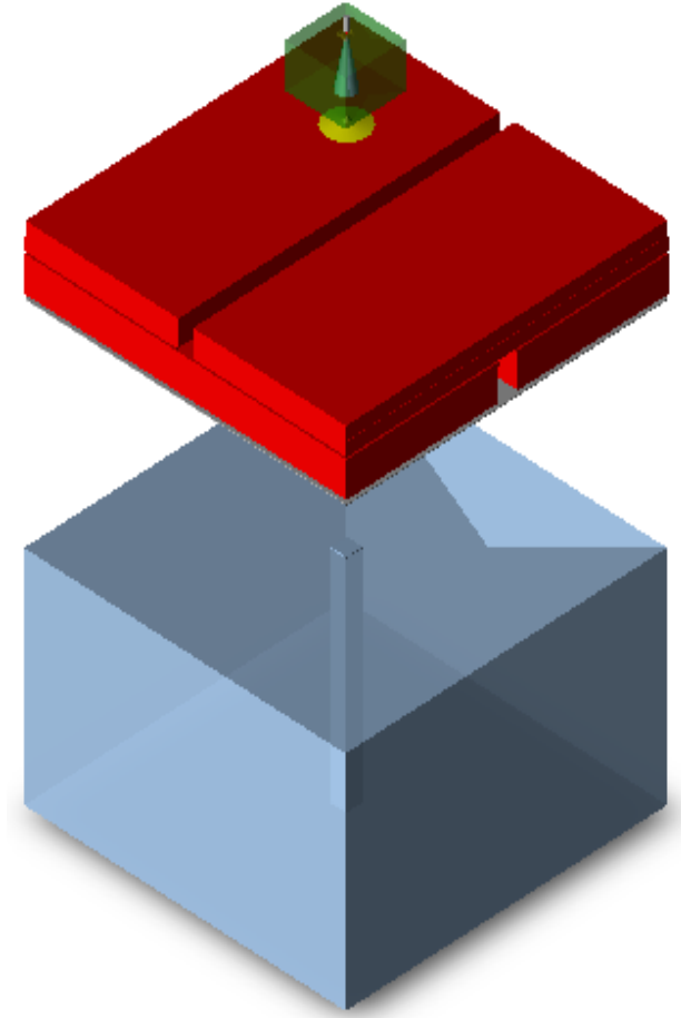
Şekil 3.4: Lineer hızlandırıcı gantry ve su fantomu modeli
