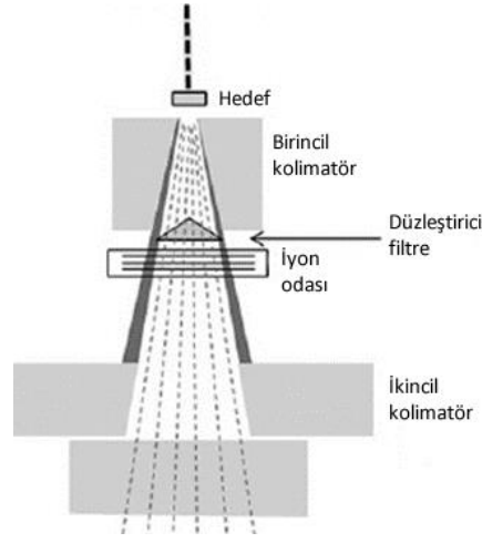
Şekil 2.17: Lineer hızlandırıcı gantry şeması 19
