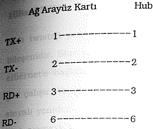
Şekil 2.11 Ağ arayüz kartı - hub kablosu pin bağlantı şeması.
