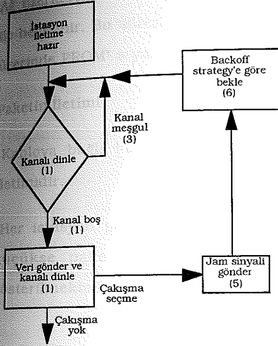
Şekil 2.8 Ethernet CSMA/CD erişim algoritması [24].
