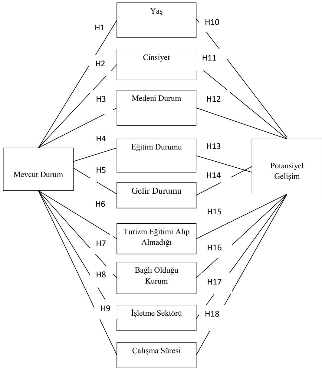
Şekil 3.1 Araştırma Modeli
