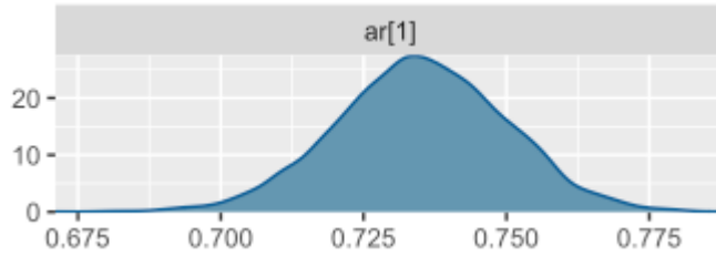
Şekil 4.16. Tahminlere ait otoregresif parametre için sonsal dağılım grafiği
