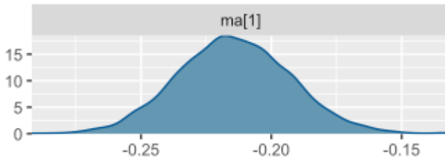
Şekil 4.17. Kalıntılara ait otoregresif parametre için sonsal dağılım grafiği
