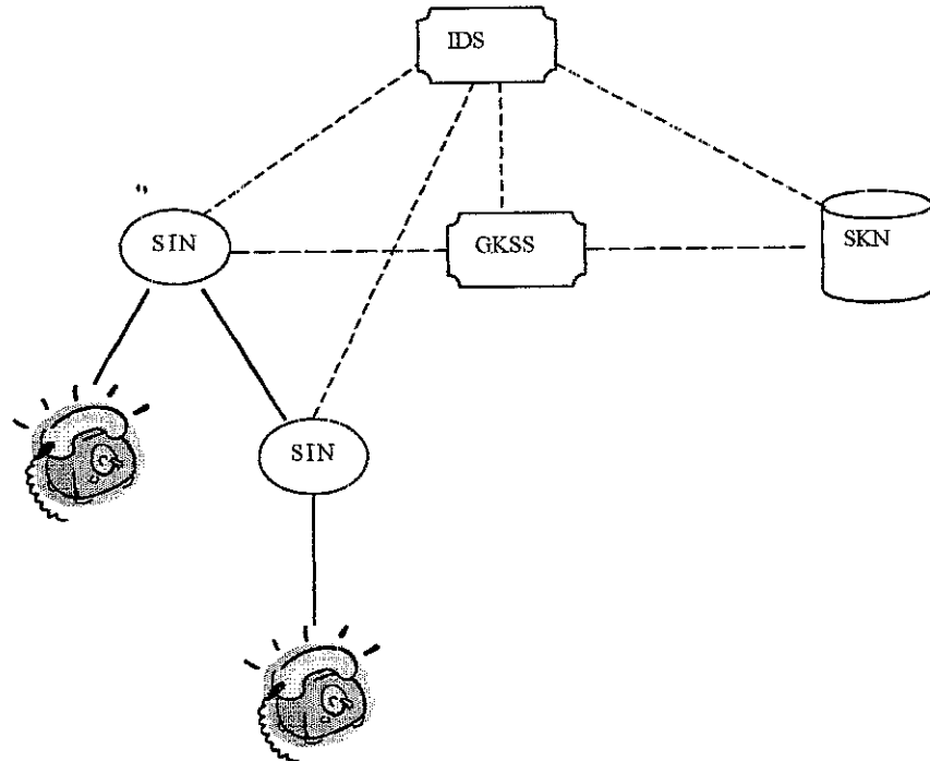
Şekil 1.6 Akıllı Şebeke
