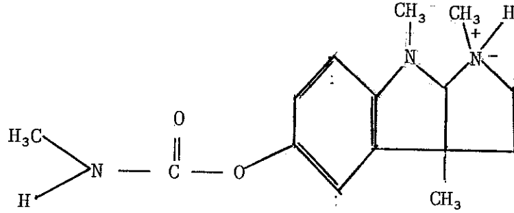
Şekil II: Fizostigmin (Eserin)
