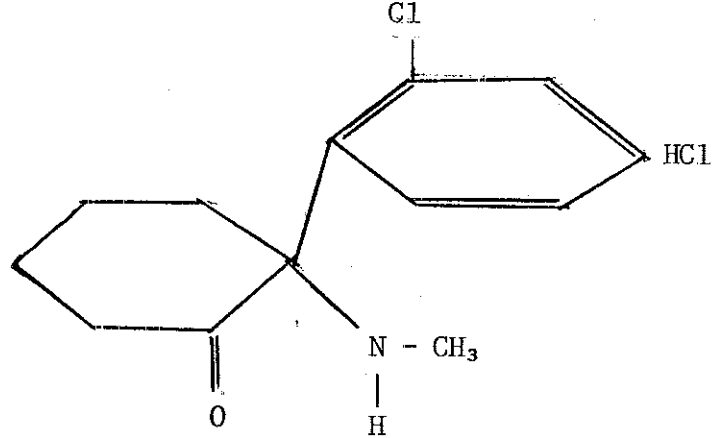
Şekil I: Ketamin Hidroklorür açık formülü 2-(0-Chlorophenyl) -2- (Methylamino) - Cyclohexanone - Hydrochloride
