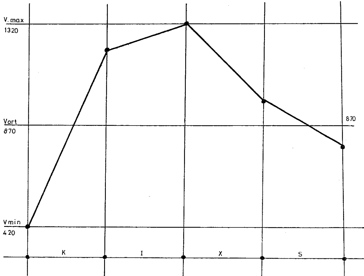
Şekil 7-5: Yukarıda istenen koşullarda Demirköprü haznesinin mevsimsel işletme politikası.
