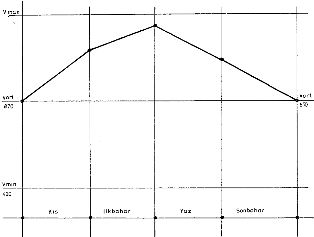
Şekil 7-2: Yukarıda istenen koşullarda Demirköprü haznesinin mevsimsel işletme politikası
