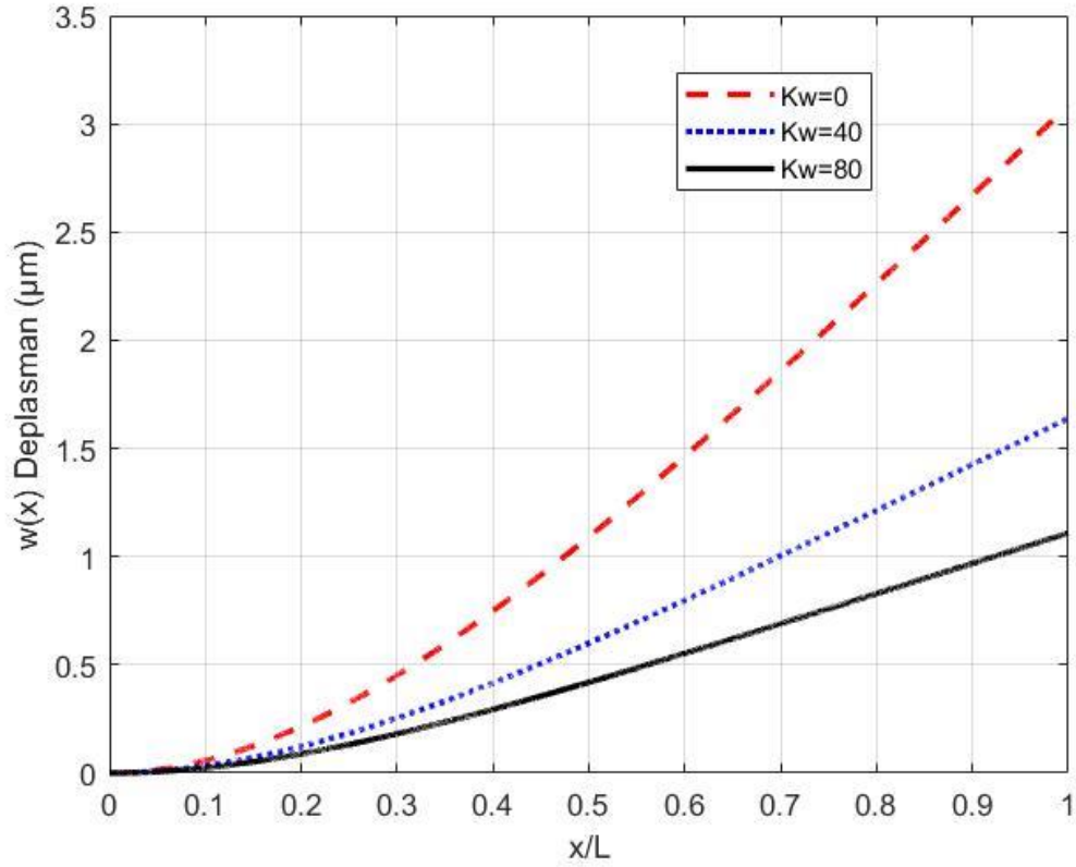
Şekil 4. 8. Boyut parametresi ( l=1,553 ) iken konsol mikro kirişin q=10\mu\text{N} yayılı yük altında x/L kiriş boyunca deplasman deplasmanın değerlerinin değişimi
